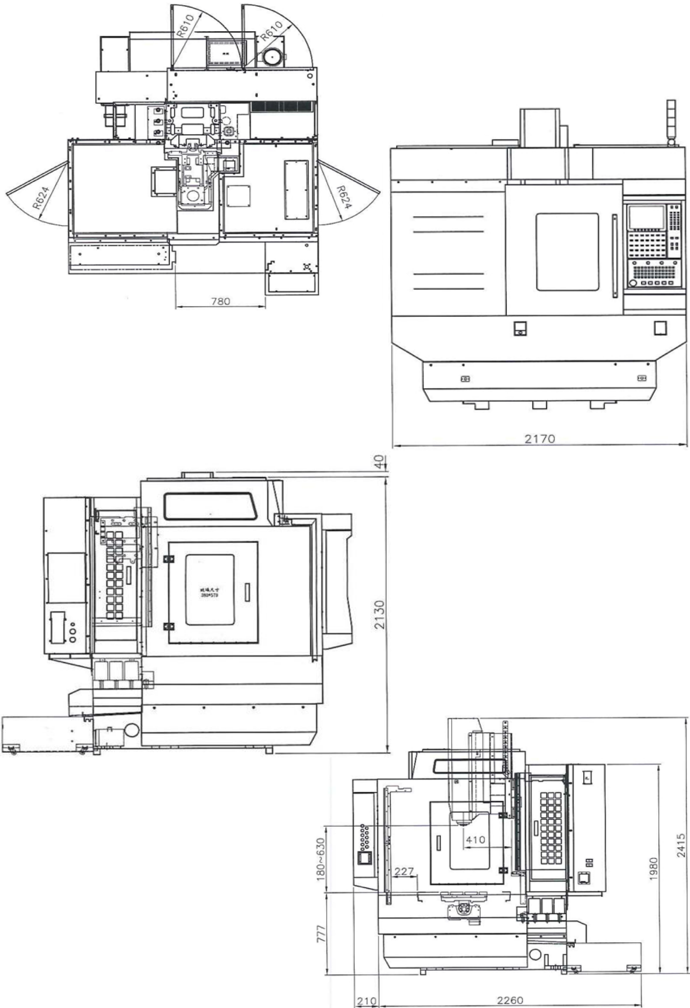
e-500.500L外型尺寸
