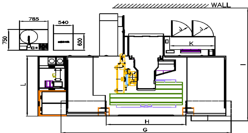
TMQ-15外型尺寸圖
